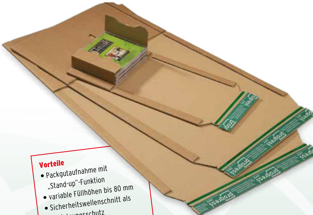
„stand-up“-Funktion durch Scharnier- rillung, schnelles Befüllen
